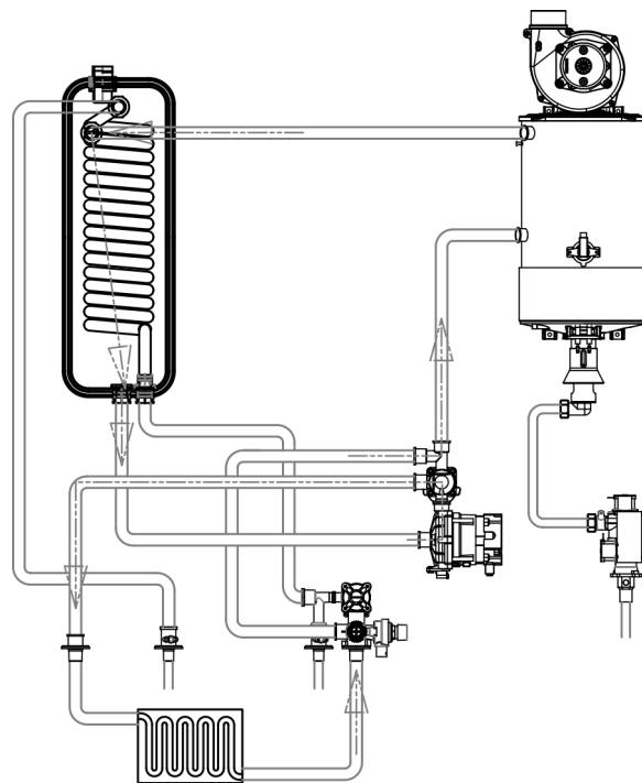
Рисунок 4. Схема работы контура отопления
