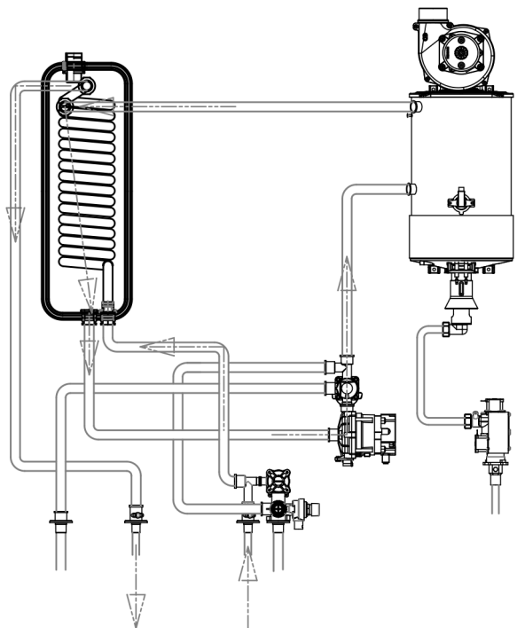
Рисунок 5. Схема работы контура ГВС
