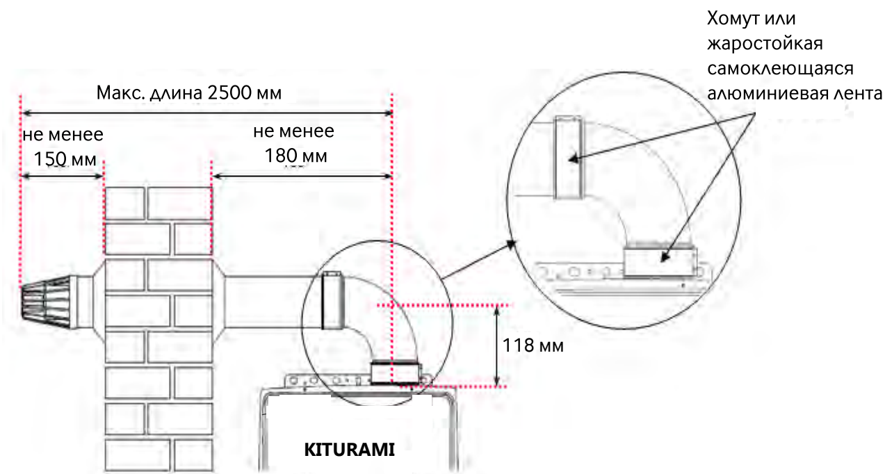
Рисунок 12. Установка дымохода
