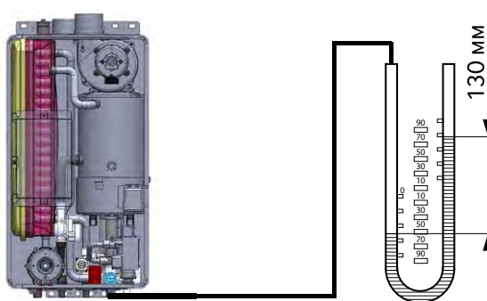
Рисунок 9. Проверка номинального давления подачи природного газа
