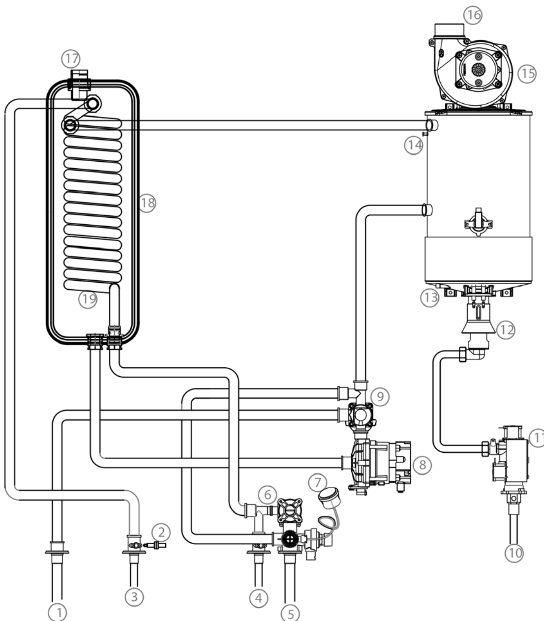
Рисунок 2. Функциональная схема котла
